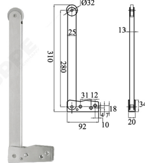
DOOR SELECTOR DEKKSON DSR 300 SSS
